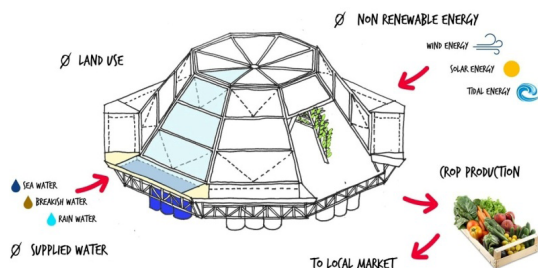
FIGURE 3. REPRÉSENTATION SCHÉMATIQUE DE LA JELLYFISH BARGE
